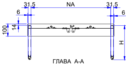
ГЛАВА А-А
